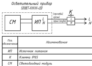
Рисунок 2 – Монтажная схема
