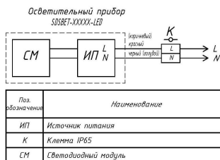
Рисунок 2 – Монтажная схема
